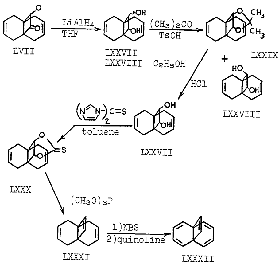
Scheme VI
