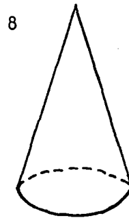
Cone
