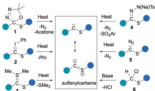
Fig. 3 Sulfenylcarbene precursors.
