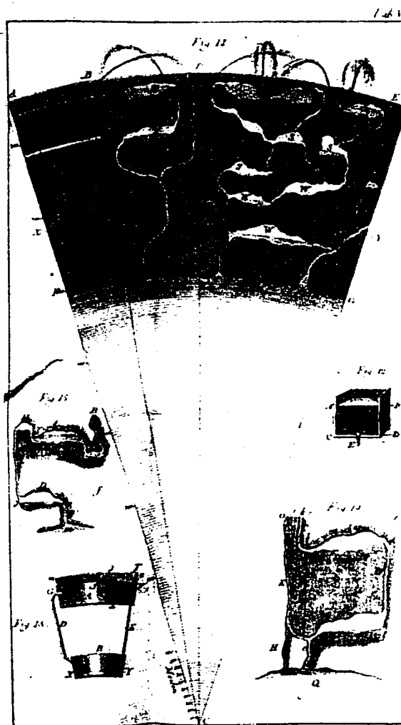
FIGURE 217. Silberschlag, Geogenie (1780), Tab V
