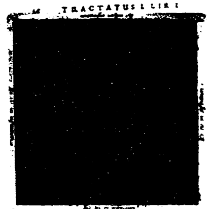
FIGURE 175. Fludd, I.1., 26. Materia prima or hyle . HSCI.
