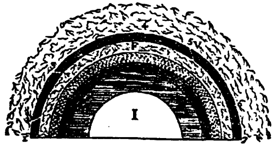
FIGURE 101. First global hemisection. Descartes, Principiae philosophiae , 1644. LH.
