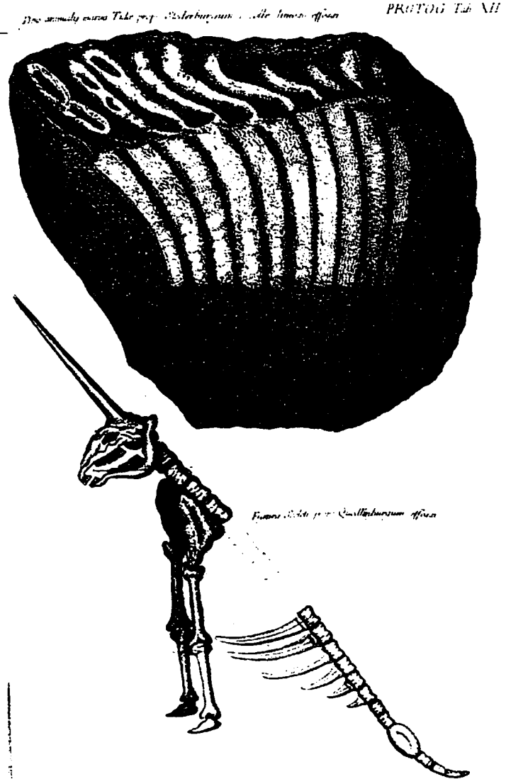
FIGURE 7. Leibniz, Protogaea (1749), Tab XII . HSCI.
