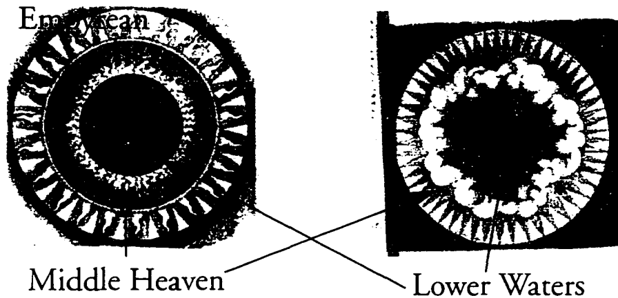
FIGURE 179. Fludd, I. II, 58. HSCI.
