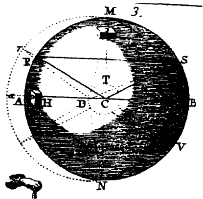
FIGURE 28. Para du Phanjas. Theoria telluris (1782). Figure 3.
