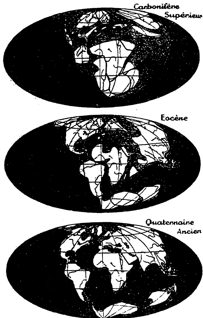
Fig. 4. — Reconstitutions du globe à trois époques géologiques d'après la théorie des translations continentales Parties hachurées : zones abyssales, parties en pointillé : mers épicontinentales. Les contours du réseau des méridiens et parallèles est arbitraire.
