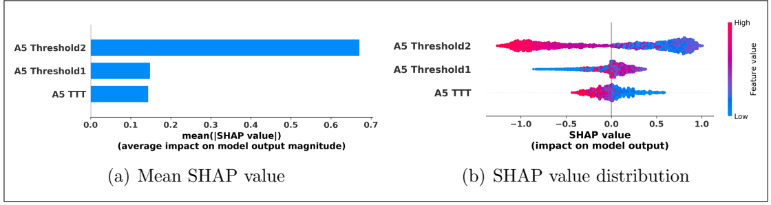
Fig. 4.1: Impact of each input parameter on RSRP
